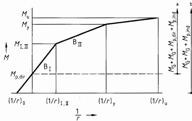
Bild 16 – Vereinfachte Momenten-Krümmungs-Beziehung für Spannbetonquerschnitte
